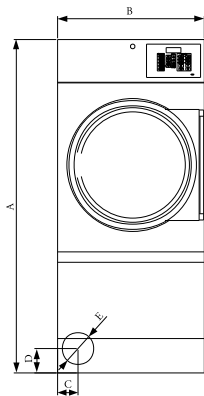
FRONT DA 11 13 15
